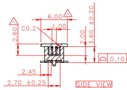
剖面圖 A-A
