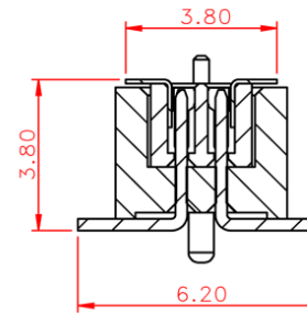
剖面圖 B-B
